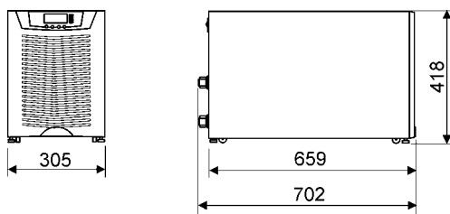
Рисунок 53. Модели ИБП без батарейных модулей
